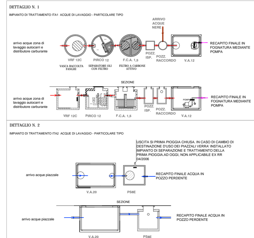
DETTAGLI - SCALA 1:100
