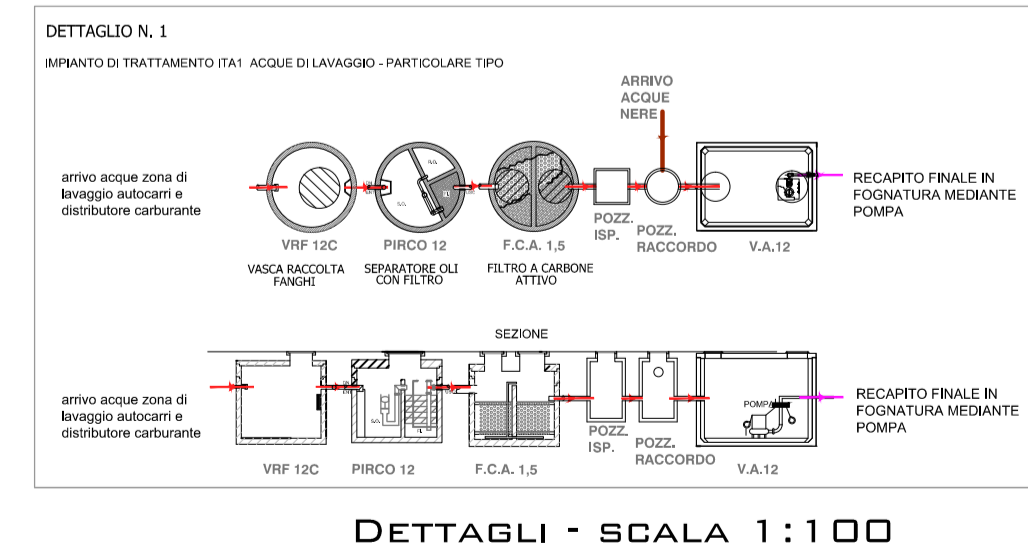
DETTAGLI - SCALA 1:100
