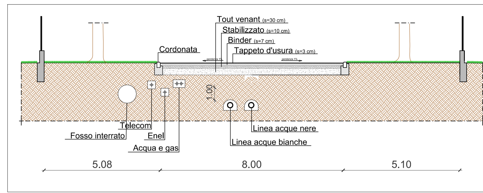
SEZIONE STRADA AA SCALA 1:100
